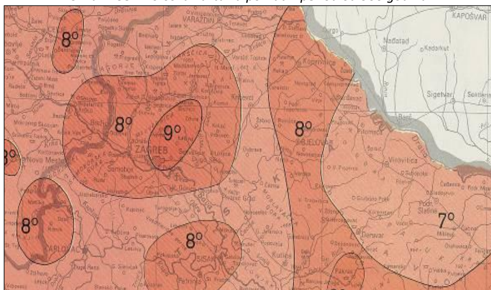
Slika 2. Seizmološka karta za povratni period od 500 godina
