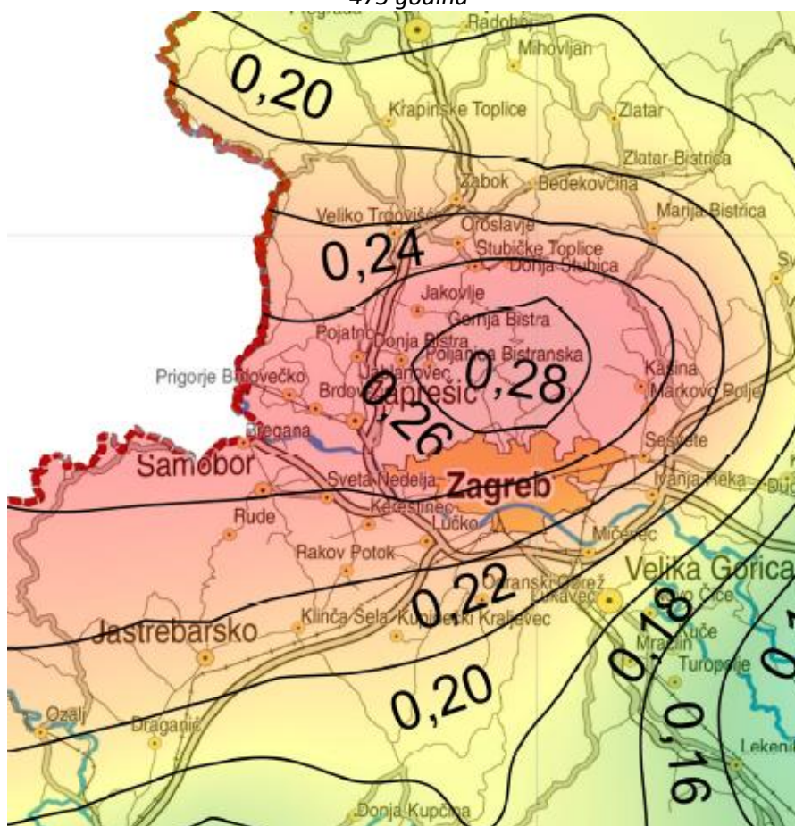
Slika 3. Vršna ubrzanja tla uzrokovana potresima za područje Grada Sveta Nedelja, za povratni period 475 godina
